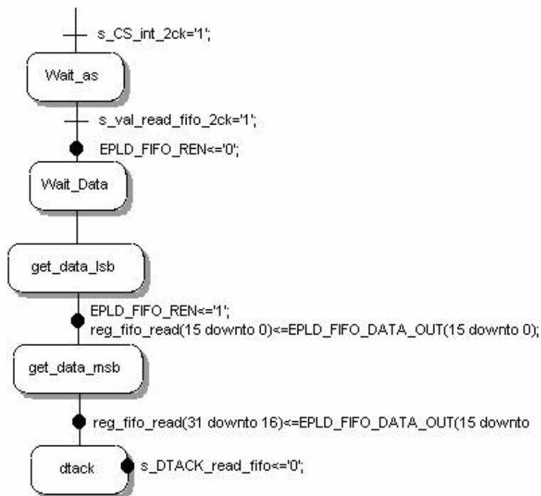
Figure 35 : FSM ReadOut
