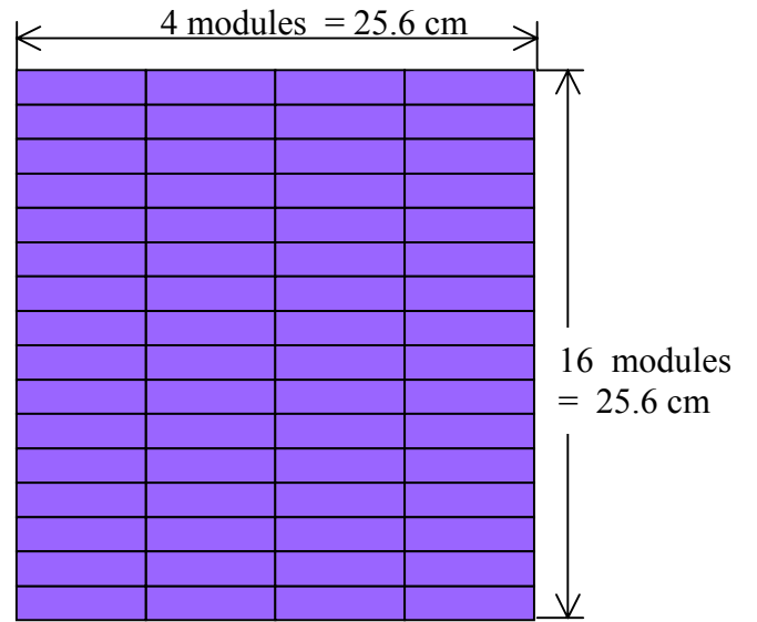
Fig. 8. Module assembly
