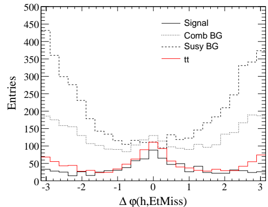
FIG. 1.3 – Distribution de l'angle dans le plan transverse à la ligne des faisceaux entre la direction de h et de E_T^{miss} , pour les événements SUSY et t\bar{t} .
