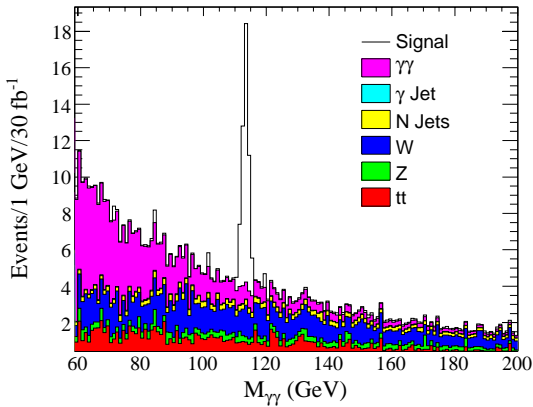
FIG. 1.4 – Distribution de la masse invariante des paires \gamma\gamma sélectionnées avec les coupures 1 et 2 du texte.
