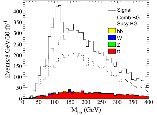
FIG. 1.2 – Distribution de la masse invariante des paires b\bar{b} sélectionnées avec les coupures 1, 2, 4 et 5 du texte.
