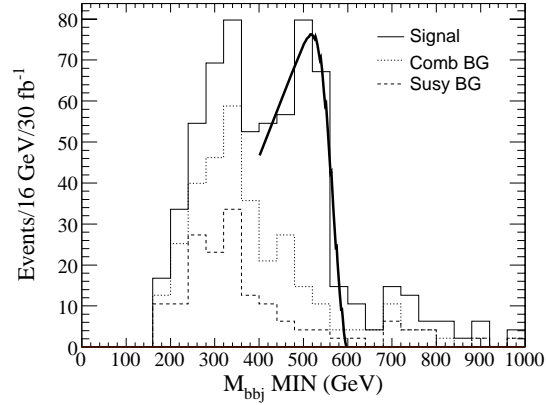
FIG. 1.5 – Distribution de la masse invariante du système b + b + q , choisis comme décrit dans le texte.
