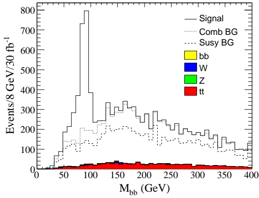
FIG. 1.1 – Distribution de la masse invariante des paires b\bar{b} sélectionnées avec les coupures 1 à 5 du texte.
