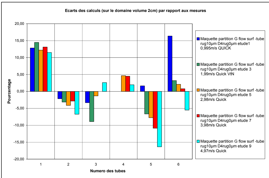
Fig. 31 Ecarts relatifs cas n°3.
