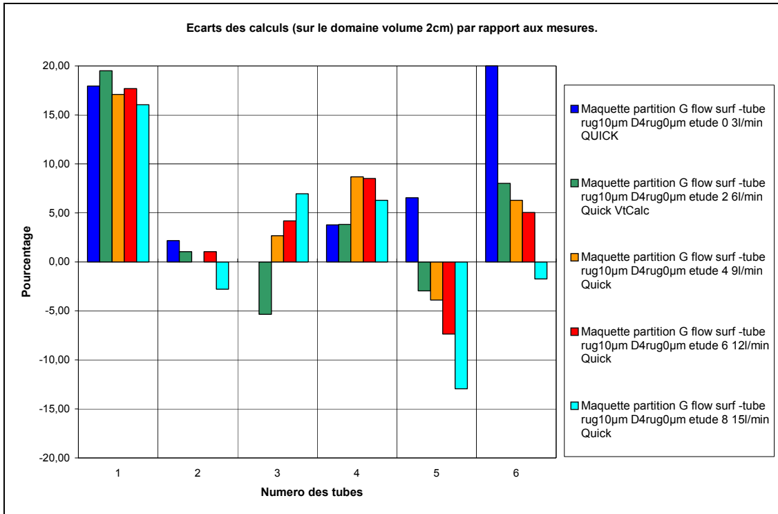
Fig. 30 Ecarts relatifs pour chaque tube entre le calcul et la mesure cas n°2.
