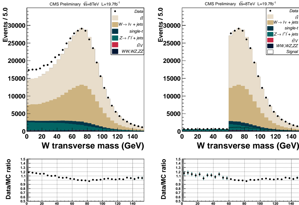
Fig. 4.10 – Distribution de la masse transverse du W avant coupure (à gauche) et après (à droite).
