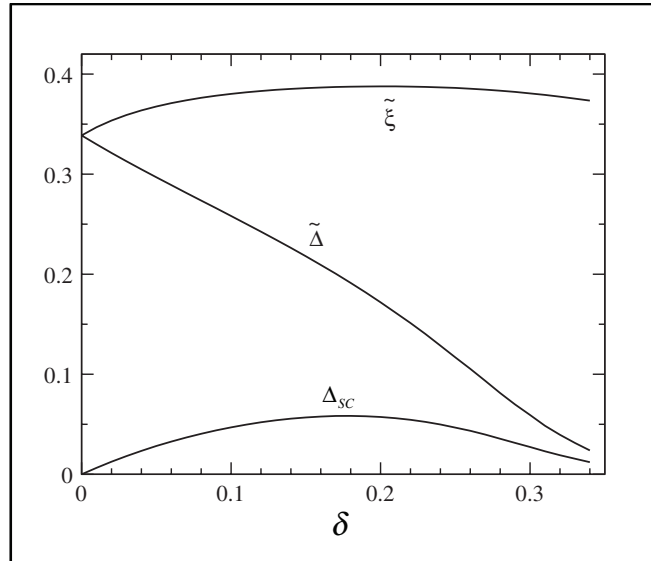
Figure 5 : Dépendance vis-à-vis du dopage \delta en trous des amplitudes de saut \tilde{\xi} = \sum_{\sigma} \langle \hat{c}_{\vec{r}\sigma}^\dagger \hat{c}_{\vec{r}\pm\vec{u}_x\sigma} \rangle_{\Phi_{d-wave}^{(BCS)}} = \sum_{\sigma} \langle \hat{c}_{\vec{r}\sigma}^\dagger \hat{c}_{\vec{r}\pm\vec{u}_y\sigma} \rangle_{\Phi_{d-wave}^{(BCS)}} et d'appariement dans le canal d'onde d \tilde{\Delta} = \langle \hat{\Delta}_{\vec{r}, \vec{r}\pm\vec{u}_x}^\dagger \rangle_{\Phi_{d-wave}^{(BCS)}} = -\langle \hat{\Delta}_{\vec{r}, \vec{r}\pm\vec{u}_y}^\dagger \rangle_{\Phi_{d-wave}^{(BCS)}} pour la fonction d'onde BCS non projetée Eq. (5). \Delta_{SC} = \langle \hat{\Delta}_{\vec{r}, \vec{r}\pm\vec{u}_x}^\dagger \rangle_{\Phi^{(RVB)}} \simeq g_t \tilde{\Delta} est une estimation du paramètre d'ordre supraconducteur dans l'état RVB associé. Ces résultats sont issus de l'approximation de champ moyen renormalisé pour le modèle t-J avec un super-échange J = t/3 . Reproduit de la référence [Ede07].
