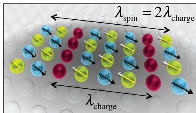
Figure 3 : Représentation schématique de « stripes » antiferromagnétiques verticales de périodes \lambda_{charge} = 4 en charge et \lambda_{spin} = 8 en spin.
