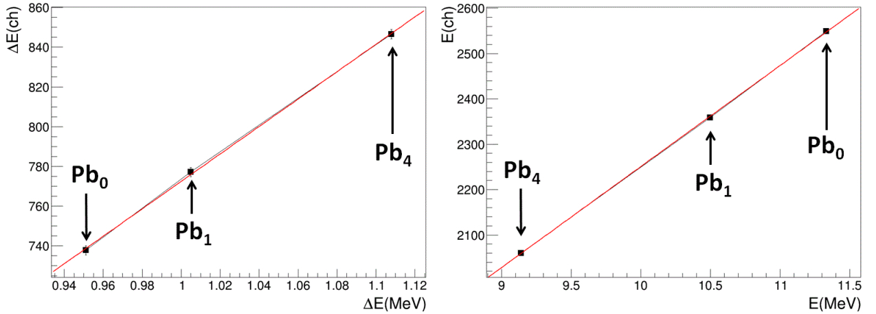
Figure D.3.: Droites de calibration de la perte d'énergie des protons dans les parties \Delta E (à gauche) et E (à droite) pour une piste \Delta E - E (à 132^\circ ) pour la réaction ^{208}\text{Pb}(d,p) . La courbe rouge correspond à un ajustement linéaire des points de calibration représentés en noir.
