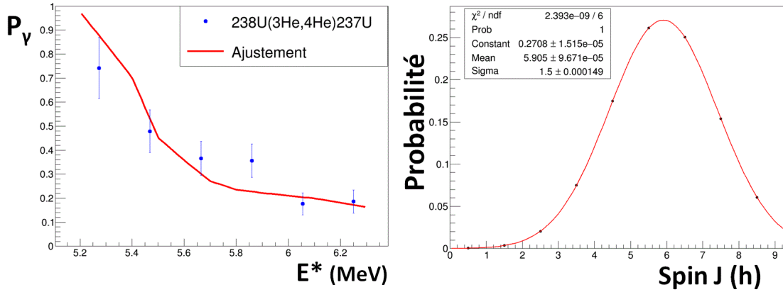
Figure E.29.: L’ajustement de P_\gamma^{\text{transfert}} à l’aide de l’équation E.10 est représenté en rouge (à gauche) pour ^{237}\text{U}^* . Distribution de spin obtenue grâce à l’ajustement de P_\gamma^{\text{transfert}} (à droite).
