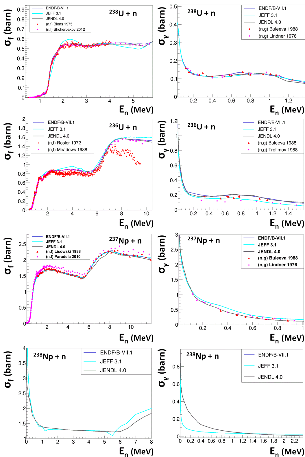
Figure E.1.: De haut en bas et de gauche à droite : sections efficaces neutroniques de fission et de capture de ^{238}\text{U} , de ^{236}\text{U} , du ^{237}\text{Np} du ^{238}\text{Np} . Les références des mesures sont indiquées dans le texte. Dans chaque cas, trois évaluations internationales ont été représentées : ENDF/B.VII.1, JEFF 3.1 et JENDL 4.0.
