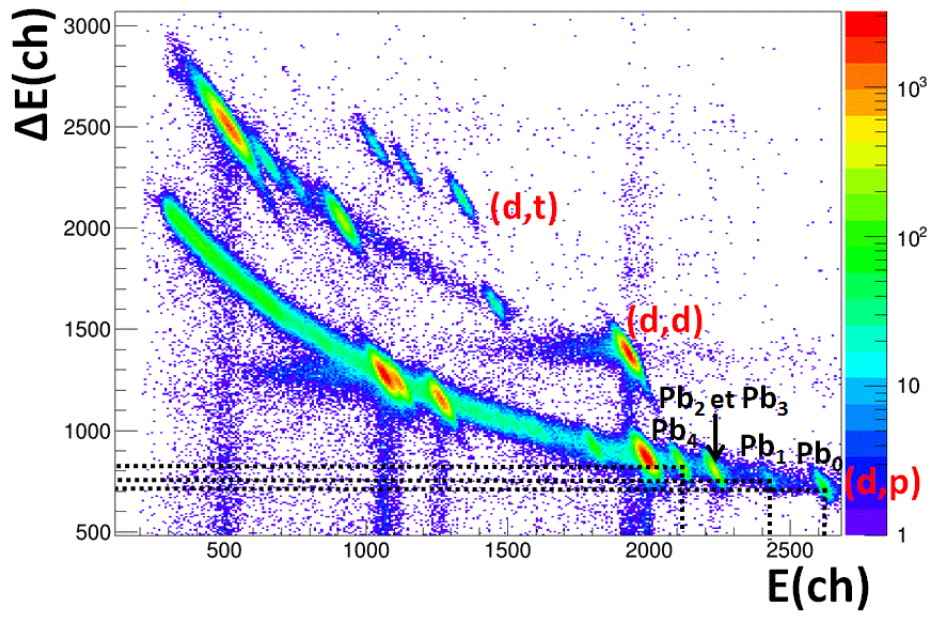
Figure D.2.: Perte d'énergie des éjectiles dans les deux parties du télescope pour une piste \Delta E-E (à 126^\circ ). Les états d'excitation du ^{209}\text{Pb} utilisés pour la calibration des SiRi sont signalés en noir. Les lignes en pointillés symbolisent la position de la valeur moyenne (en canaux) de la perte d'énergie des protons provenant des états Pb_0 , Pb_1 et Pb_4 dans les parties E et \Delta E de la piste du télescope.
