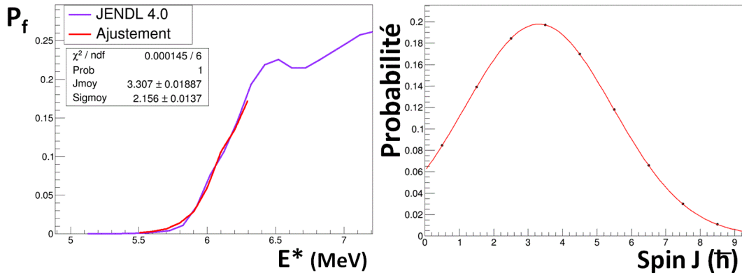
Figure E.25.: L'ajustement de P_f^{JENDL} pour 1^{237}\text{U}^* à partir de l'équation E.10 est représenté en rouge (à gauche). Distribution de spin obtenue grâce à l'ajustement de P_f^{JENDL} sur la gamme énergétique [5,6-6,3 MeV] (à droite).
