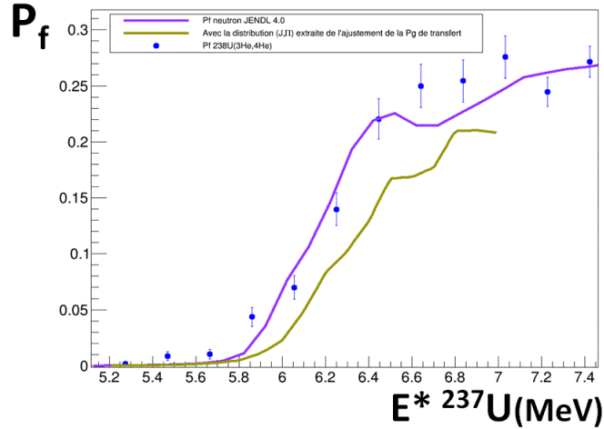
Figure E.30.: Probabilité de fission de l' ^{237}\text{U}^* obtenue avec la distribution de spin extraite du fit de P_{\gamma}^{transfert} en comparaison avec la probabilité neutronique donnée par JENDL 4.0 et les données expérimentales obtenues avec la réaction U(^{2383}\text{He}, ^4\text{He}) .
