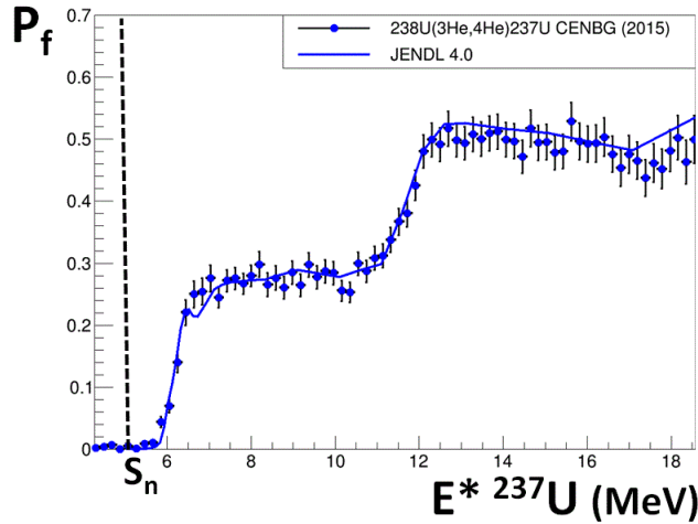
Figure E.20.: Probabilité de fission de ^{237}\text{U}^* en fonction de l'énergie d'excitation comparée à l'évaluation JENDL 4.0.
