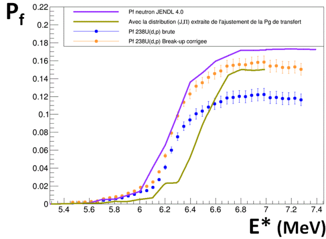
Figure E.19.: Probabilité de fission de l' ^{239}\text{U}^* obtenue avec la distribution de spin extraite de l'ajustement de P_\gamma^{transfert} dans la gamme énergétique [S_n-6,3 \text{ MeV}] en comparaison avec la probabilité neutronique donnée par JENDL 4.0 et les données expérimentales obtenues avec la réaction (d,p) non corrigées, et corrigées du break-up.
