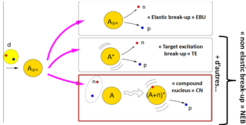
Figure E.4.: Illustration du mécanisme de quelques processus de break-up du deuteron approchant un noyau cible A. La composante recherchée correspond à la formation du noyau composé et est encadrée en rouge.
