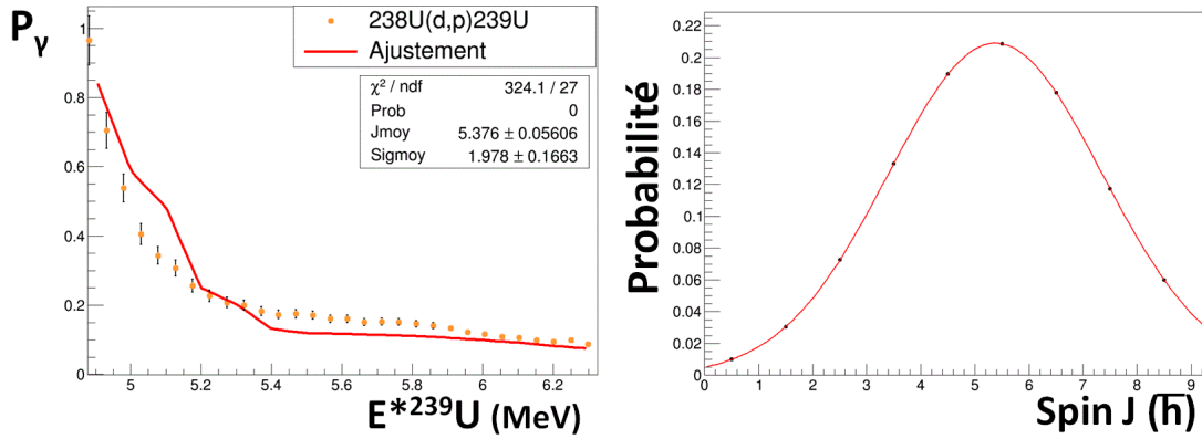
Figure E.18.: L’ajustement de P_{\gamma}^{transfert} à partir de l’équation E.10 est représenté en rouge (à gauche). Distribution de spin obtenue grâce à l’ajustement de P_{\gamma}^{transfert} sur la gamme énergétique [S_n-6,3 \text{ MeV}] (à droite).
