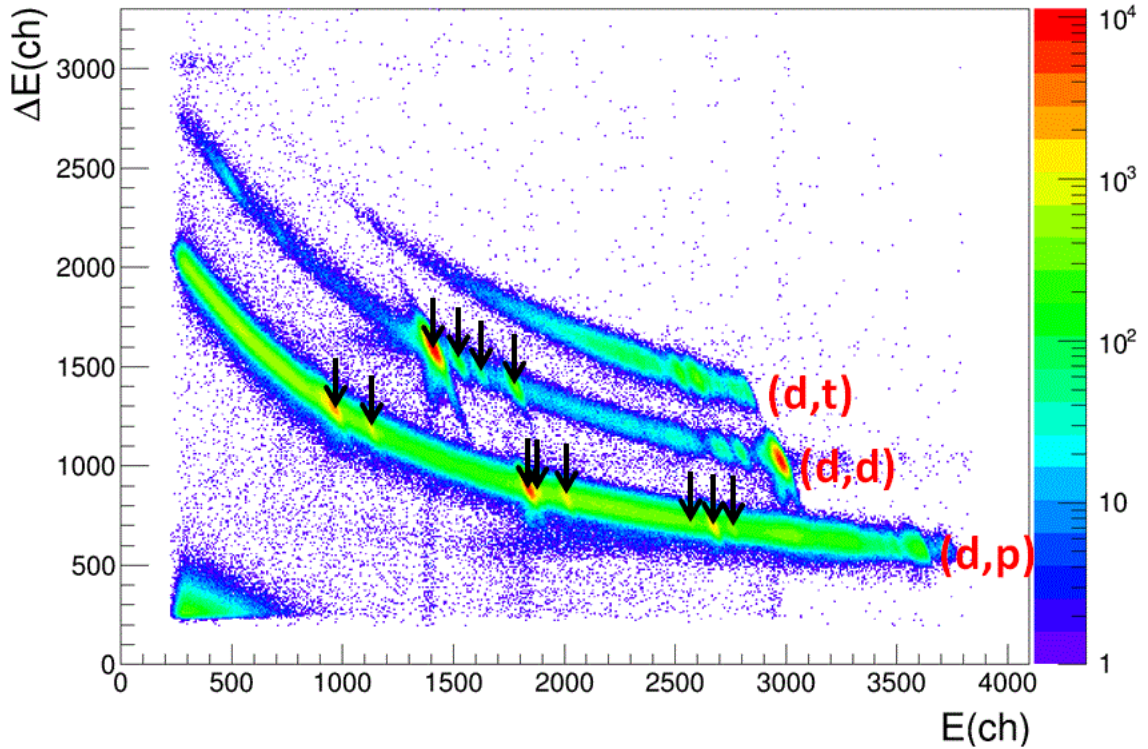
Figure D.1.: Perte d'énergie des éjectiles dans les deux parties du télescope pour une piste \Delta E-E (à 126^\circ ). Les flèches noires signalent la présence d'une contamination au carbone ou à l'oxygène.
