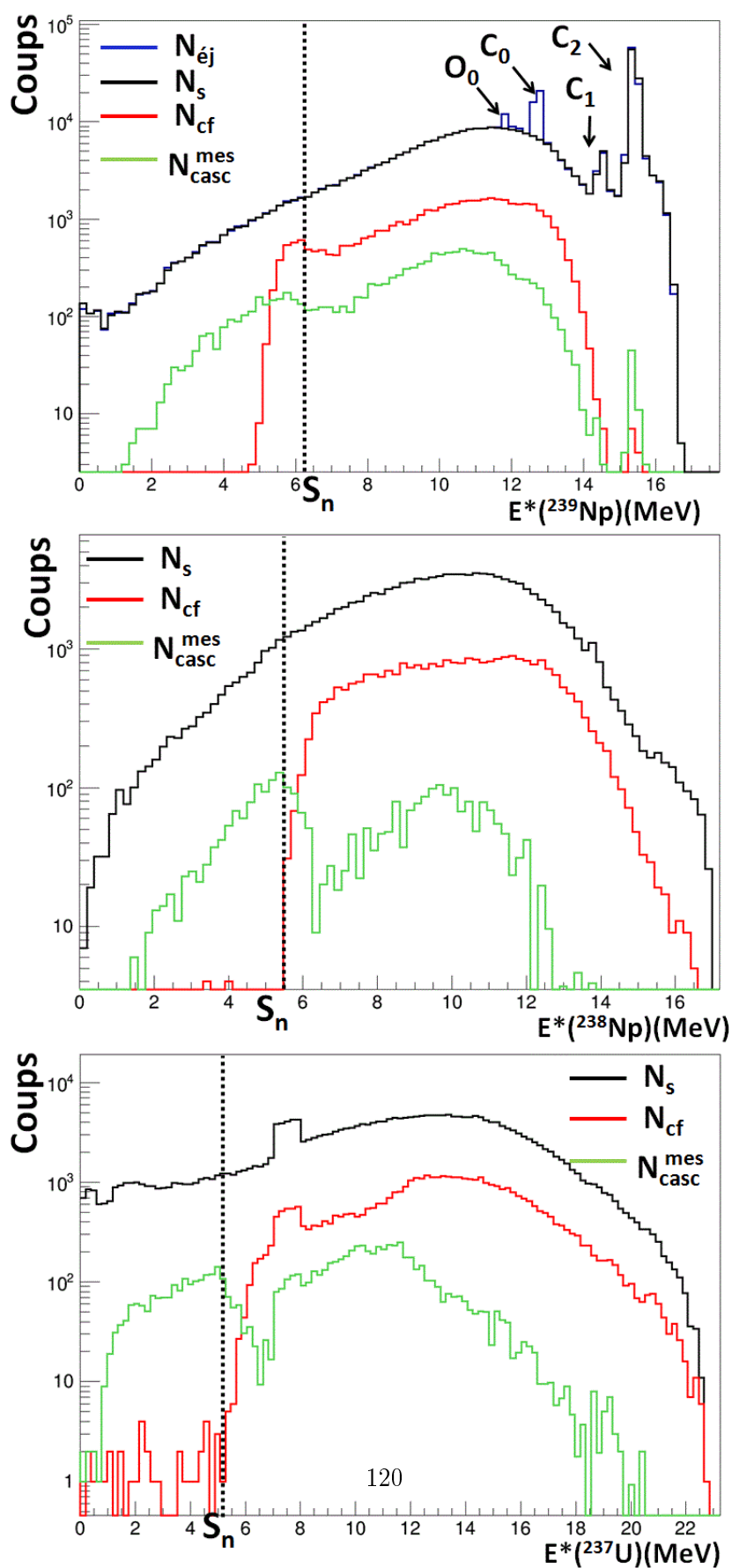
Figure D.27.: Spectres singles N_s(E^*) , de coïncidences fission N_{cf}(E^*) et de coïncidences gammas N_{casc}^{\text{mes}}(E^*) pour les noyaux composés ^{237}\text{U} , ^{238}\text{Np} et ^{239}\text{Np} . La ligne en pointillé représente l'énergie de séparation du neutron.
