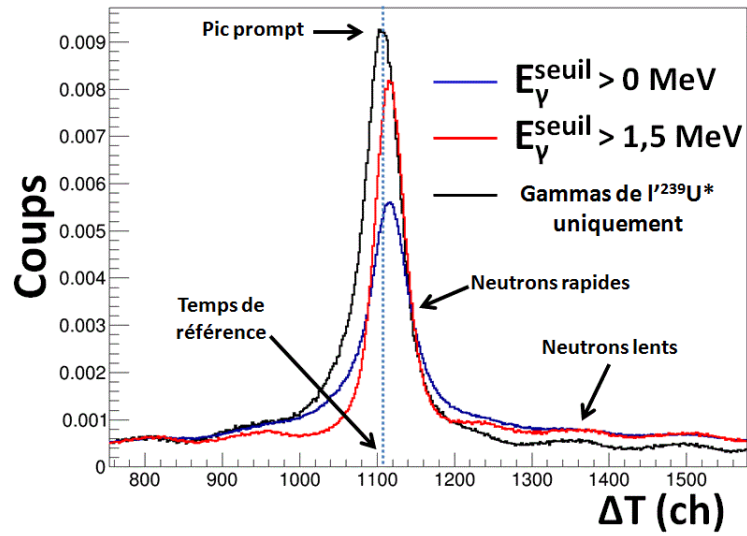
Figure D.19.: Proportion d'évènements détectés (normalisée à 1) en fonction de la différence en temps. La courbe noire ne concerne que les gammas émis par 1^{239}\text{U}^* d'énergie d'excitation inférieure au S_n , alors que les courbes rouge et bleue incluent également la contribution due aux neutrons détectés pour différents seuils de détection en énergie. Le temps de coïncidence de référence correspond au maximum du pic gamma prompt et est symbolé par la ligne en pointillée.
