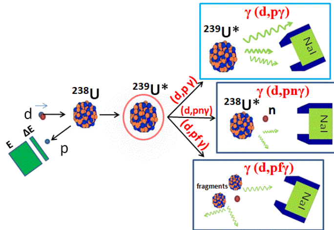
Figure D.15.: Illustration des différents modes de provenance des gammas détectés en coïncidence avec les éjectiles pour la réaction ^{238}\text{U}(d, p) .
