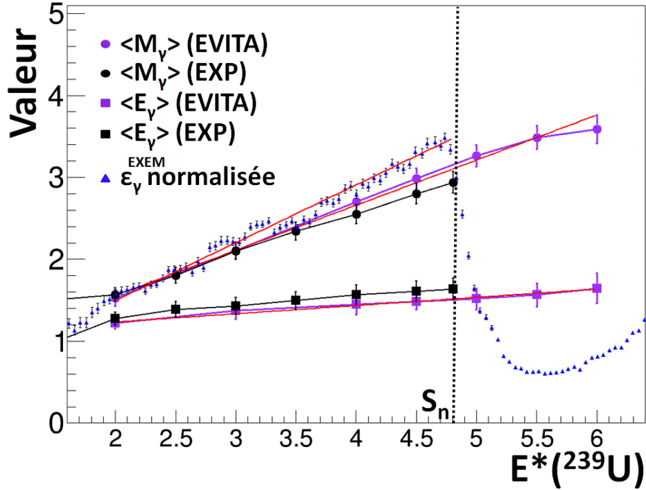
Figure D.37.: Comparaison des multiplicités et énergies moyennes des gammas émis pour des noyaux d' ^{239}\text{U}^* à différentes énergies d'excitation pour la somme des pistes à 126^\circ avec les résultats du code Monte Carlo basé sur le modèle statistique EVITA. Les lignes rouges correspondent à des ajustements linéaires. Les triangles bleus représentent l'efficacité gamma normalisée à la valeur de la multiplicité moyenne pour E^* = 2 MeV.
