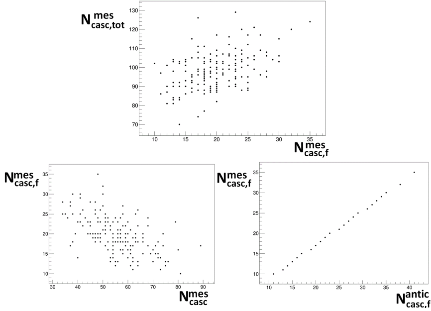
Figure D.40.: Représentation de N_{casc,tot}^{mes} = f(N_{casc,f}^{mes}) , N_{casc,f}^{mes} = f(N_{casc}^{mes}) et N_{casc,f}^{mes} = f(N_{casc,f}^{antic}) pour la réaction ^{238}\text{U}(^3\text{He}, ^4\text{He}) .
