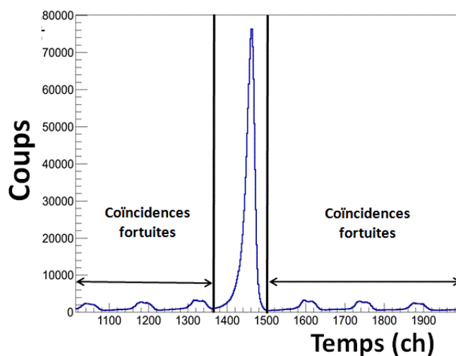
Figure D.13.: Nombre d'évènements en fonction de la différence de temps entre le télescope (start) et un fragment détecté par un des PPACs (stop) pour la réaction ^{238}\text{U}(d,p) . Les lignes noires verticales délimitent la fenêtre en temps du pic de coïncidence.
