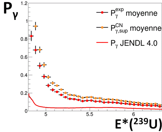
Figure E.7.: Probabilité d'émission gamma expérimentale P_\gamma^{\text{exp}} et limite supérieure de la probabilité P_{\gamma,\text{sup}}^{\text{CN}} corrigée du break-up du deuteron pour l' ^{239}\text{U}^* , comparées à la probabilité induite par neutron selon JENDL 4.0.
