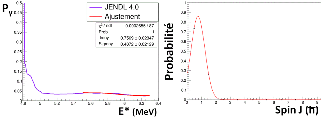
Figure E.12.: L'ajustement de P_\gamma^{JENDL} à l'aide de l'équation E.10 est représenté en rouge (à gauche). Distribution de spin obtenue grâce à l'ajustement de P_\gamma^{JENDL} sur la gamme énergétique [5,5-6,3 MeV] (à droite).
