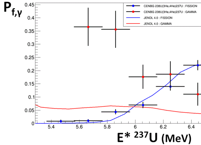
Figure E.22.: Probabilités de fission et d'émission gamma de ^{237}\text{U}^* comparées aux données évaluées dans une région énergétique commune.
