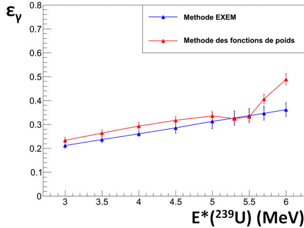
Figure D.38.: Comparaison des efficacités d'émission gamma à 126^\circ de ^{239}\text{U}^* pour différentes E^*(^{239}\text{U}) obtenues avec les méthodes des fonctions de poids et EXEM. S_n(^{239}\text{U}) = 4,806 MeV.
