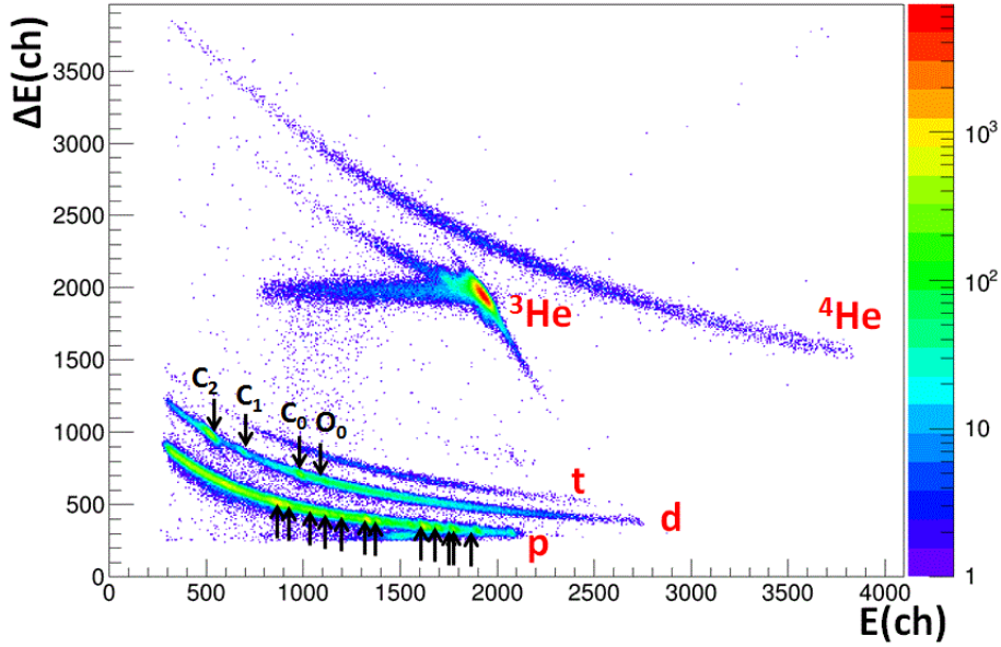
Figure D.25.: Perte d'énergie des éjectiles dans les deux parties du télescope \Delta E - E pour une piste (à 126^\circ ) impliquant le faisceau d' {}^3\text{He} et la cible d' {}^{238}\text{U} . Les flèches noires signalent la présence d'une contamination venant de la réaction sur un noyau léger de {}^{12}\text{C} , {}^{13}\text{C} ou {}^{16}\text{O} .
