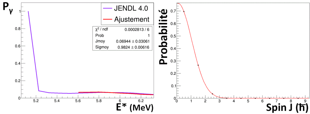
Figure E.24.: L'ajustement de P_\gamma^{JENDL} pour 1^{237}\text{U}^* à partir de l'équation E.10 est représenté en rouge (à gauche). Distribution de spin obtenue grâce à l'ajustement de P_\gamma^{JENDL} sur la gamme énergétique [5,6-6,3 MeV] (à droite).
