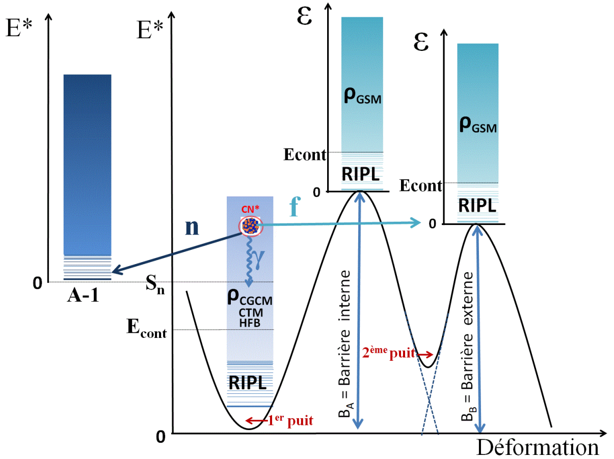
Figure A.8.: Illustration des voies de désexcitation accessibles pour un noyau composé non fissile. Le noyau composé CN se désexcite par émission gamma \gamma , émission neutron n ou par fission f . La fission est représentée par une barrière à deux bosses. A faible énergie d'excitation, la densité de niveaux \rho est définie selon les niveaux discrets de RIPL [RIPL]. A partir d'une certaine énergie, et selon l'état de déformation du noyau, \rho peut être modélisée de différentes manières (la signification des indices est indiquée dans le texte).
